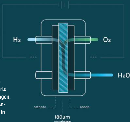
Current PEM electrolyser
